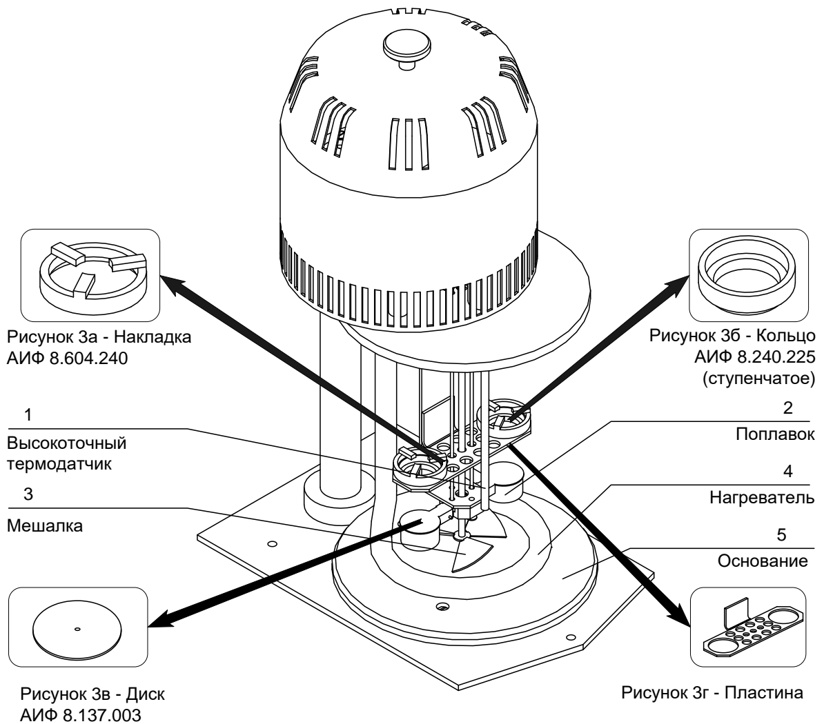
Рисунок 3 – Технологический блок
